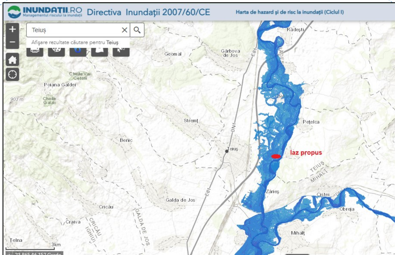
Fig. 4.5 Harta de hazard și risc la inundații
