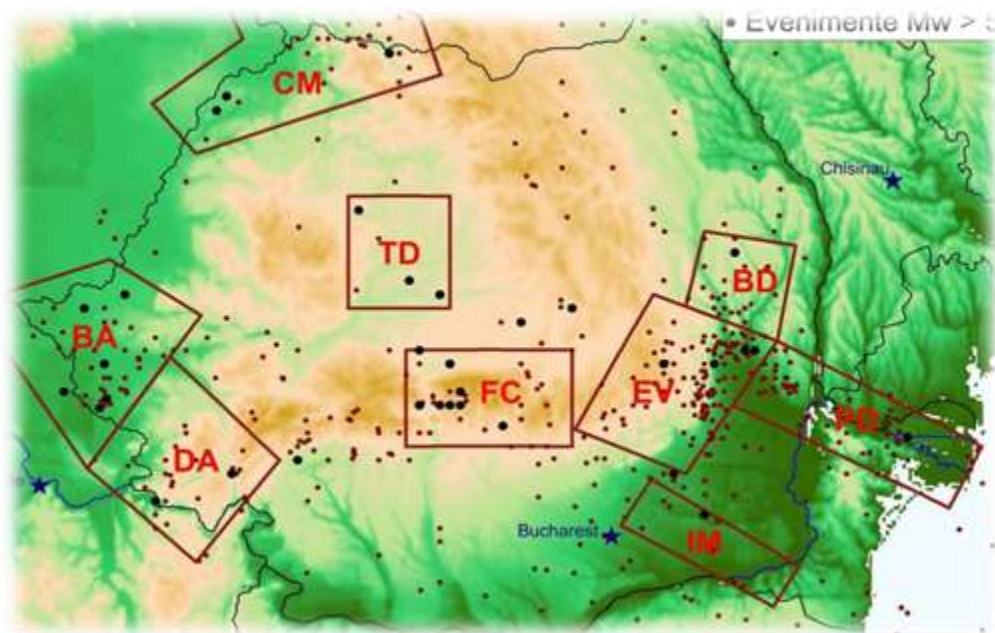
Fig. Zonele seismice din România
