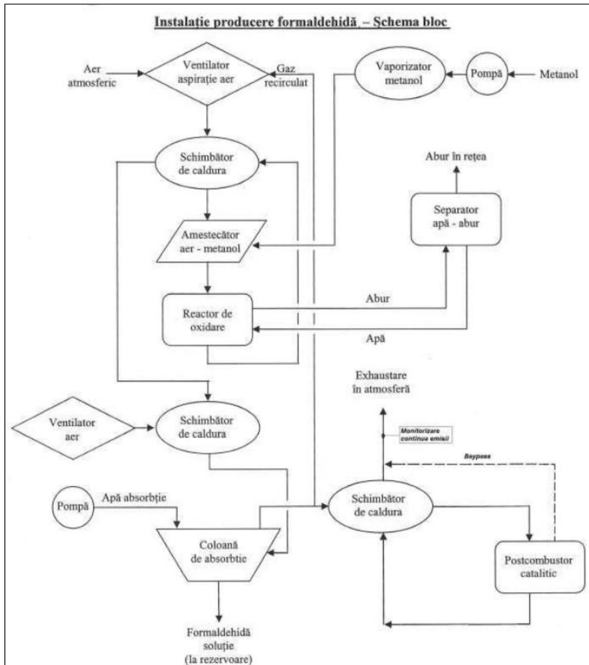
Figura nr. 2 Schema bloc a instalatiei producere formaldehida
