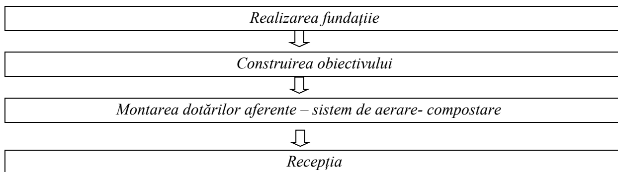
Fig.2.3 Etape procesului tehnologic de construire a halei pentru compostare
