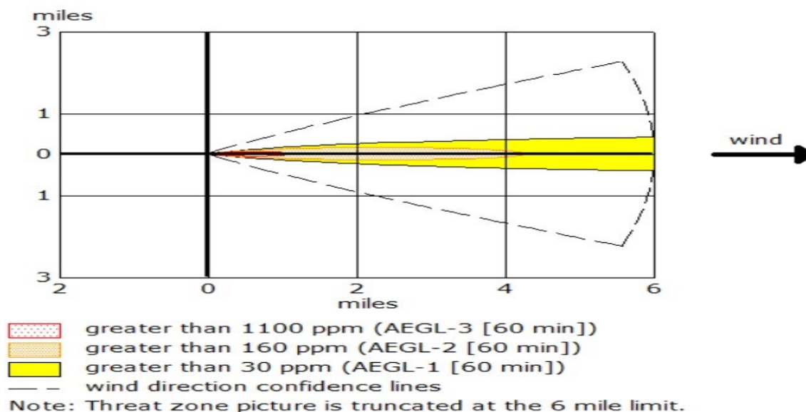
Fig. 5.3 Dispersia amoniacului
