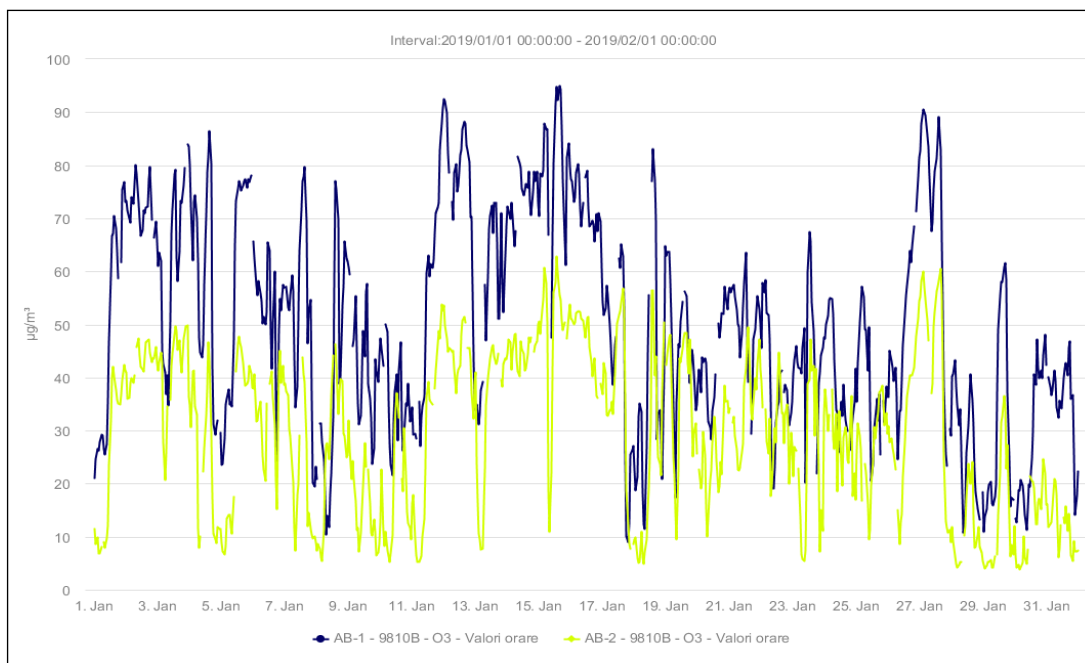
Figura. 1.1.4.1 Ozon – valori orare
