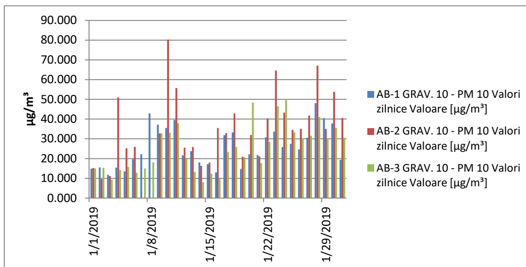
Figura. 1.1.6.2 Pulberi în suspensie PM 10 – metoda gravimetrică
