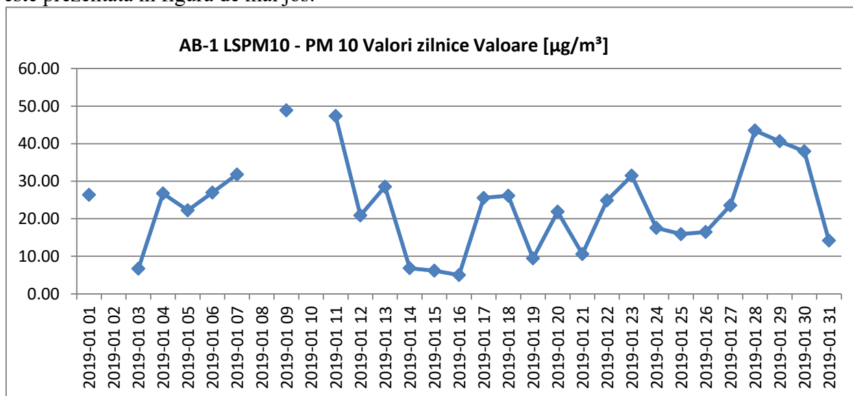
Figura. 1.1.6.1 Pulberi în suspensie PM 10 – metoda automată
