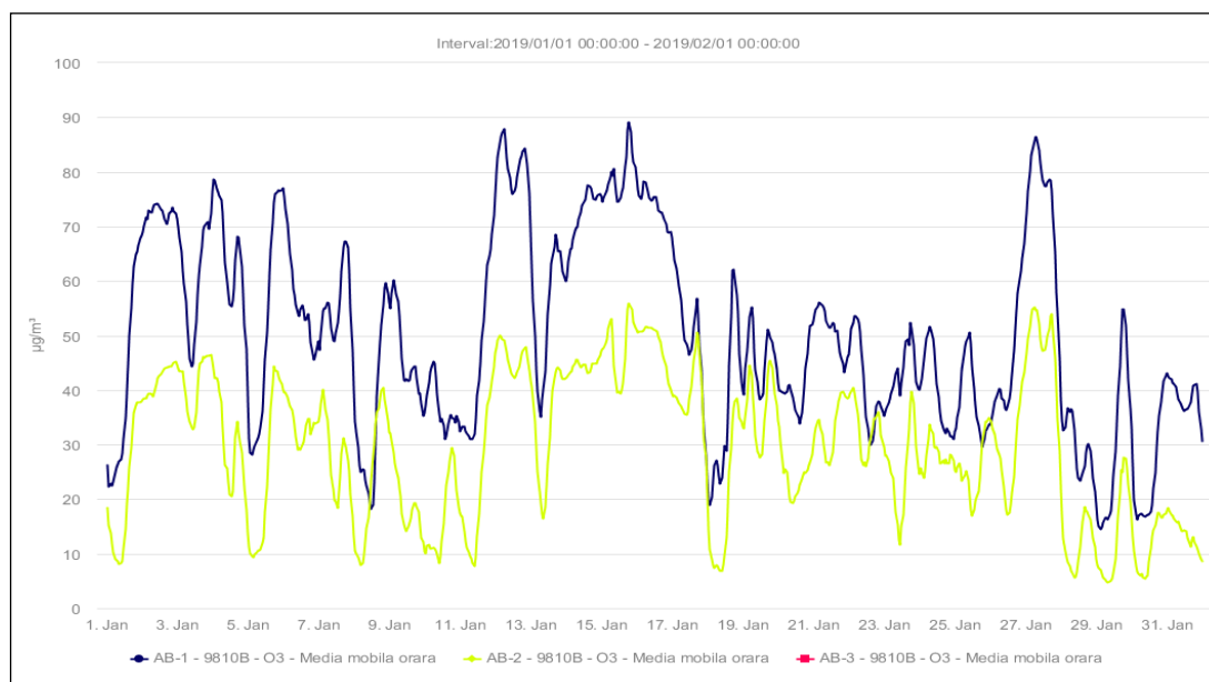
Figura. 1.1.4.2 Ozon – medie mobilă
