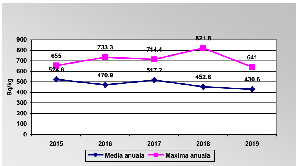
Fig. X.1.3.1-Variația mediilor și maximelor anuale ale activității specifice beta globale a solului necultivat în ultimii 5 ani(Bq/kg)
