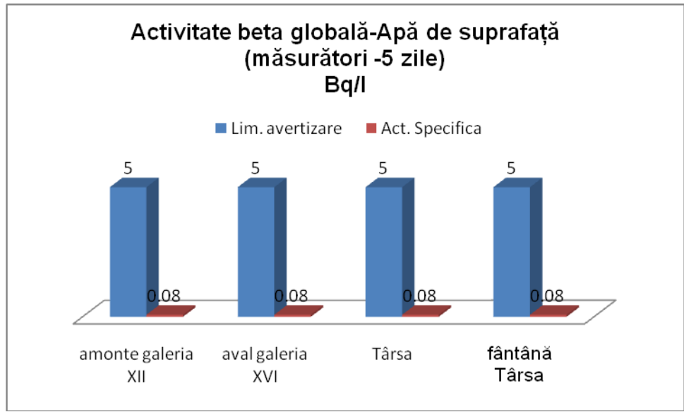
Fig. X.2.2.1-Activitate beta globală – Apă de suprafață (măsurători 5 zile)
