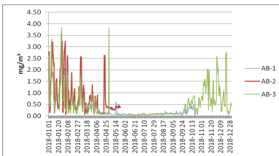
Figura nr. 6 Monoxid de carbon - Media mobilă – Date validate
