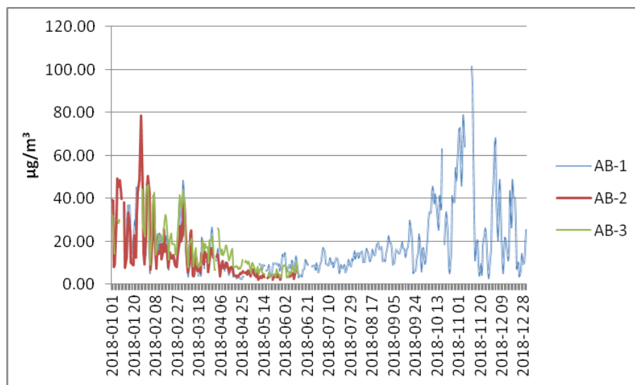
Figura nr. 4 Pulberi în suspensie PM 10 – automat
