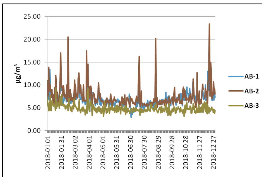
Figura nr. 3 Dioxid de sulf - Valori zilnice – Date validate
