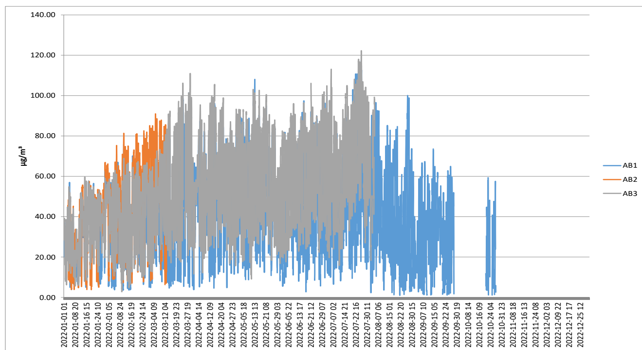
Figura nr. 7 Ozon - Valori orare – Date validate
