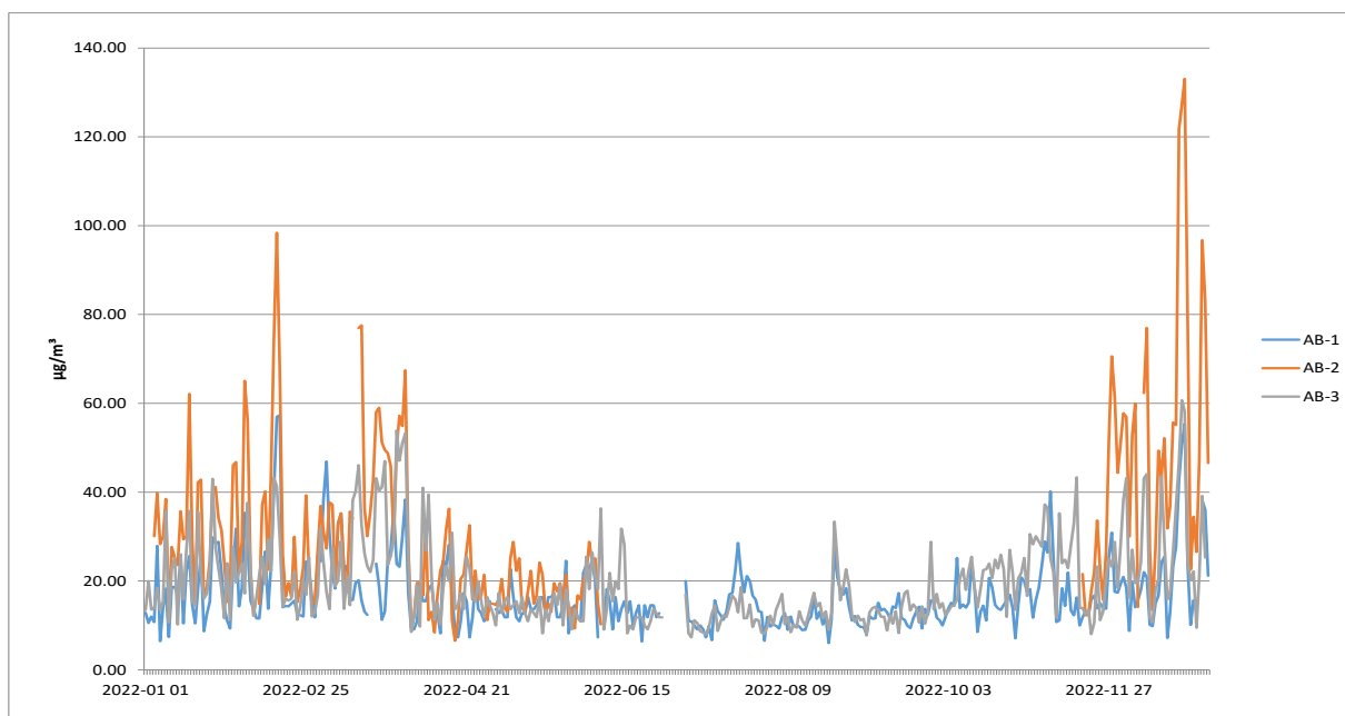
Figura nr. 5 Pulberi în suspensie PM 10 – gravimetric
