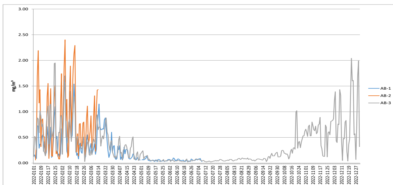
Figura nr. 6 Monoxid de carbon - Media mobilă – Date validate
