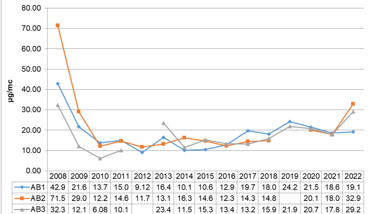
Evoluția calității aerului la indicatorul PM10 automat - medie anuală
