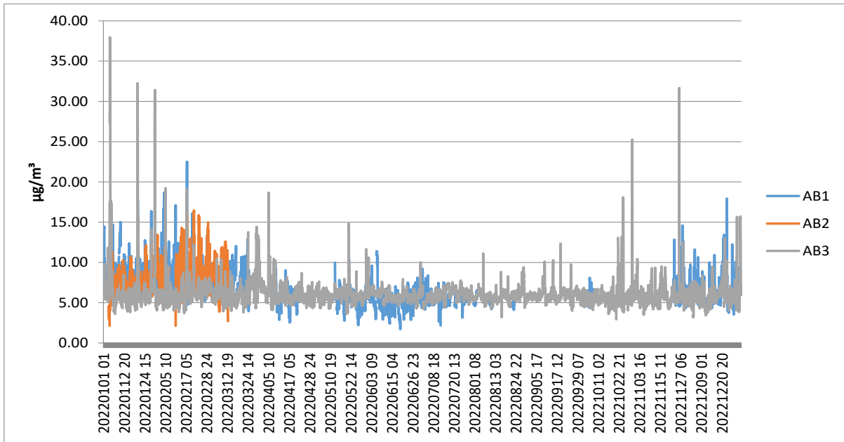
Figura nr. 2 Dioxid de sulf - Valori orare – Date validate
