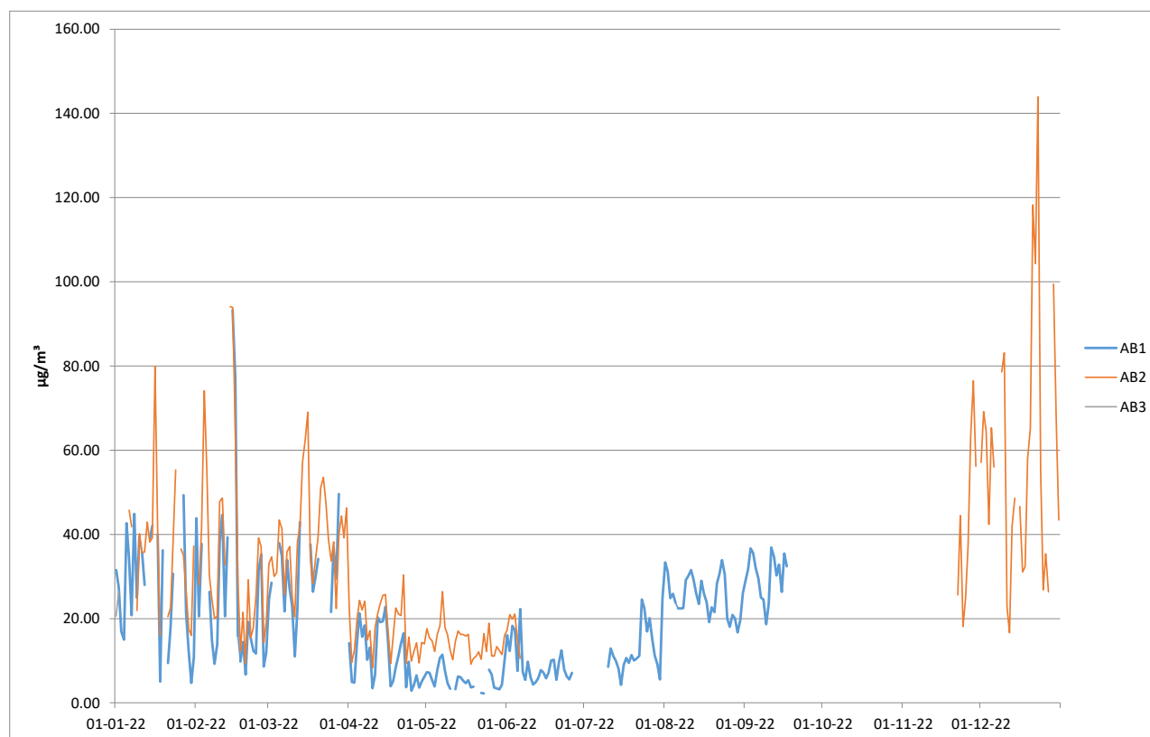
Figura nr. 4 Pulberi în suspensie PM 10 – automat
