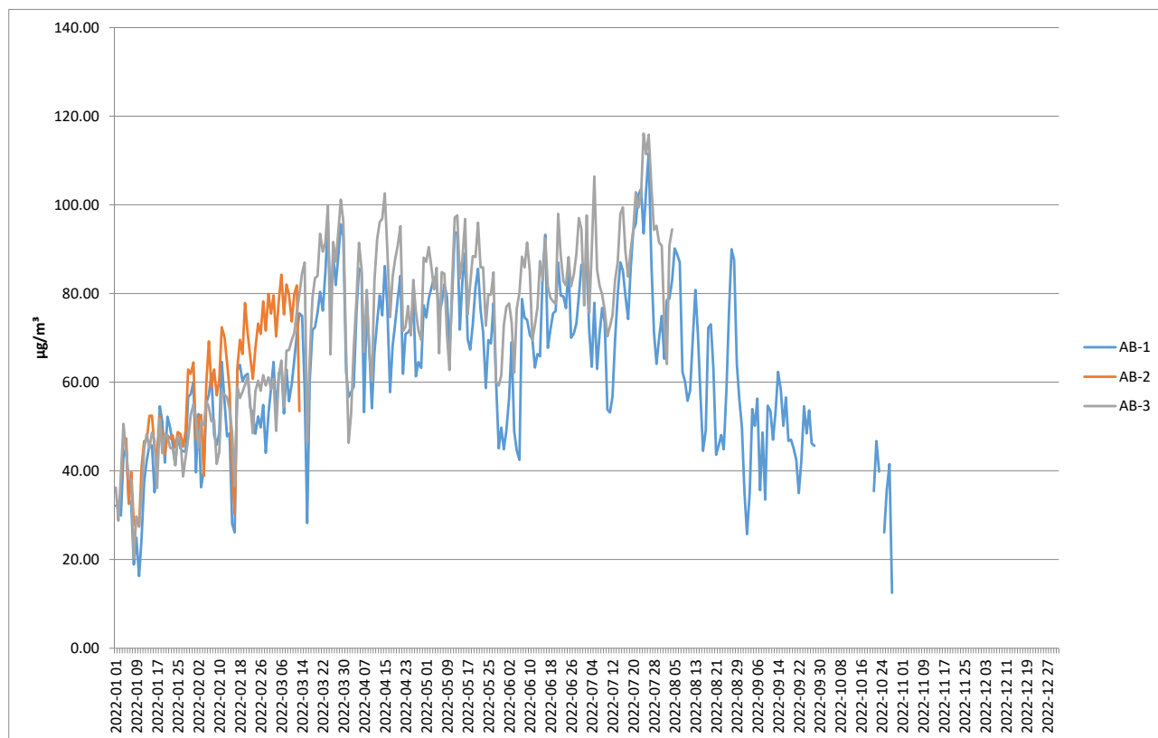
Figura nr. 8 Ozon - Media mobilă – Date validate
