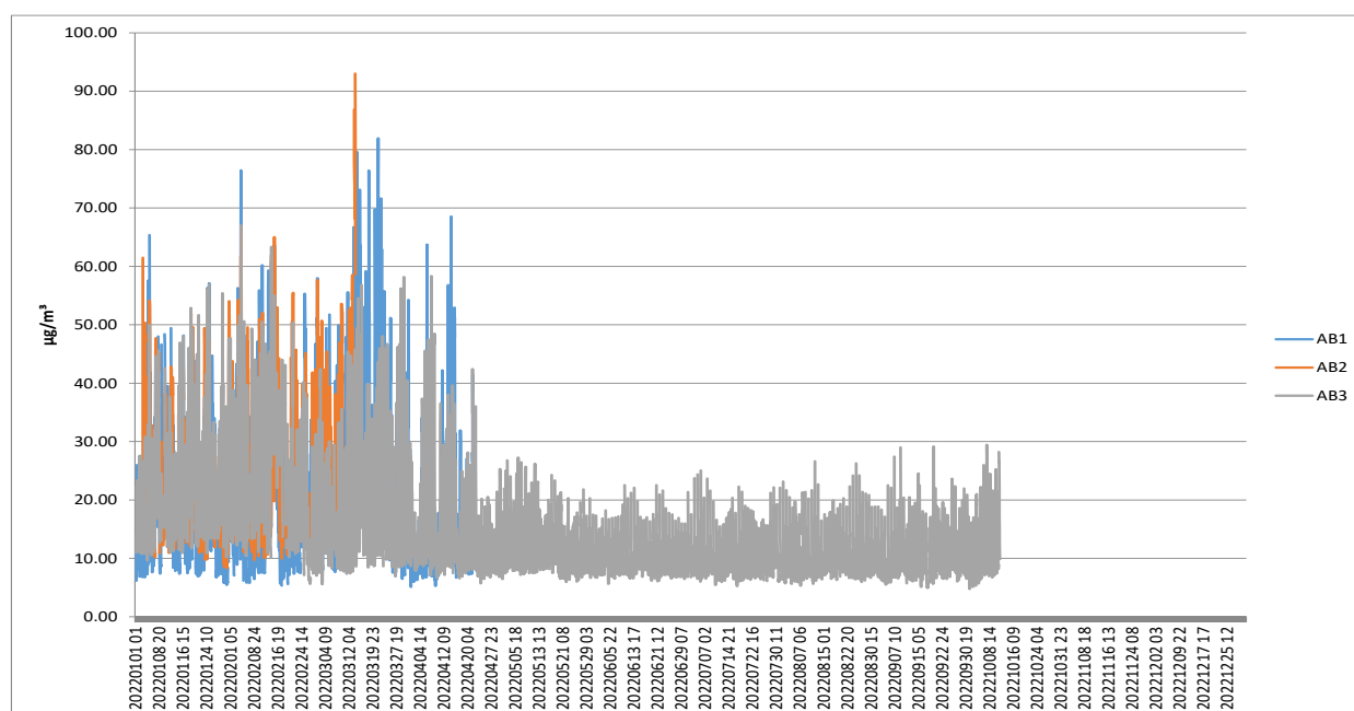
Figura nr. 1 Dioxid de azot - Valori orare - Date validate
